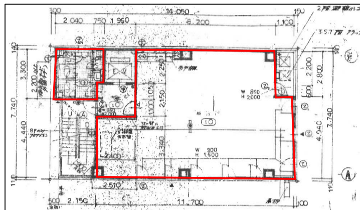
平面図
